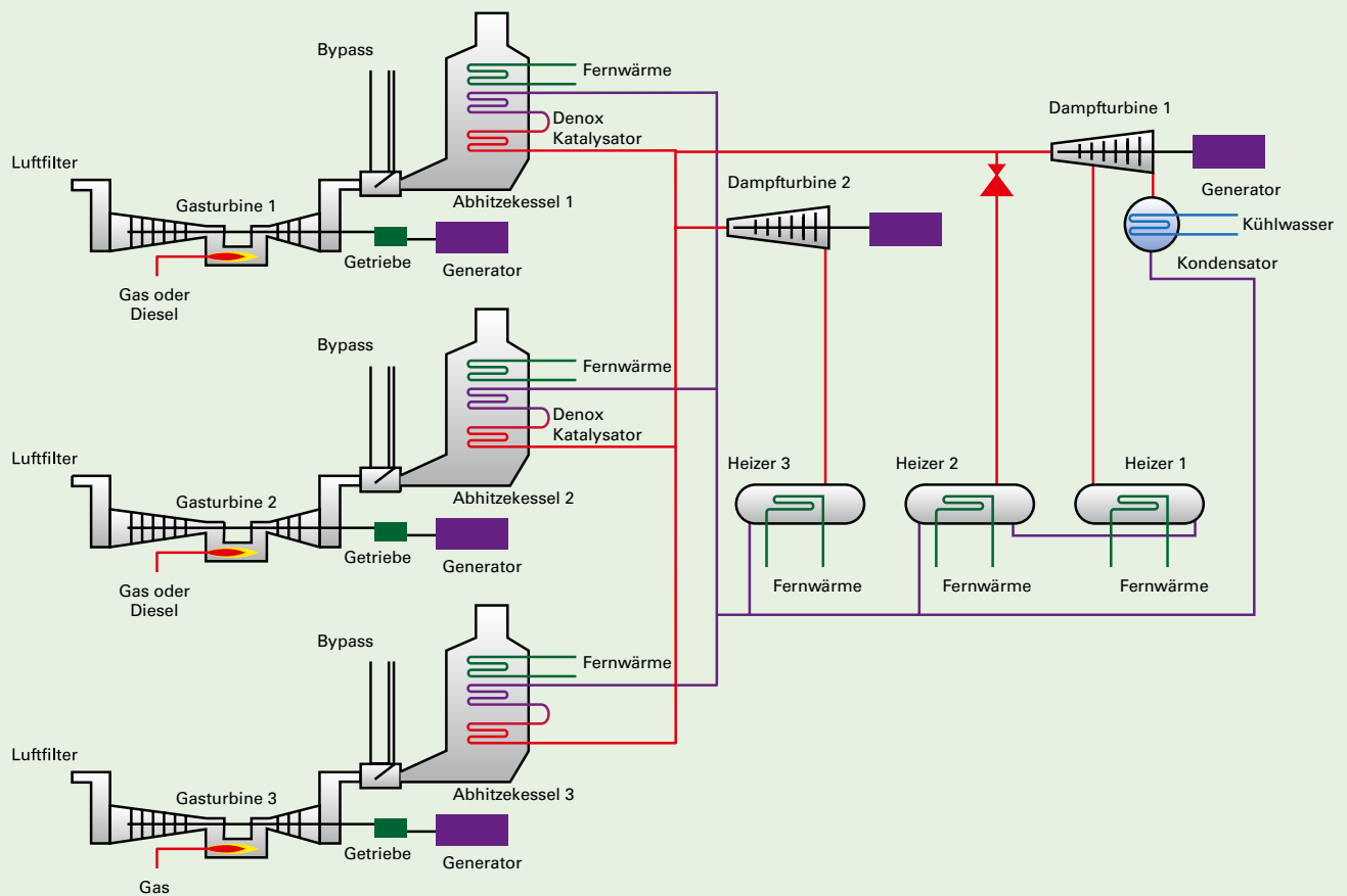
Energiepark Linz-Süd
